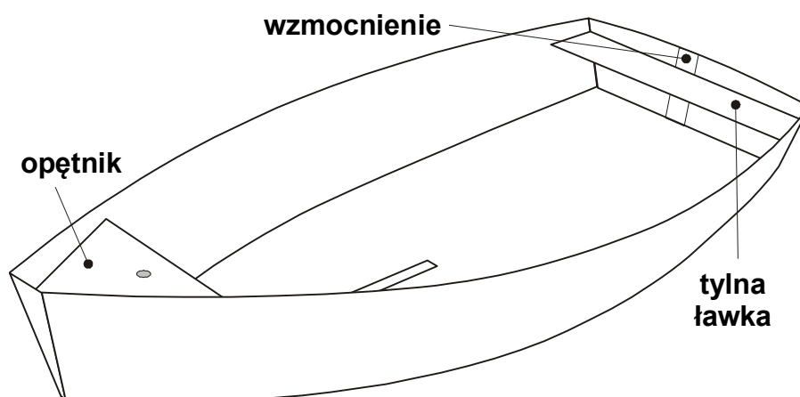
Widok kadłuba po wykonaniu pkt. 2.9
